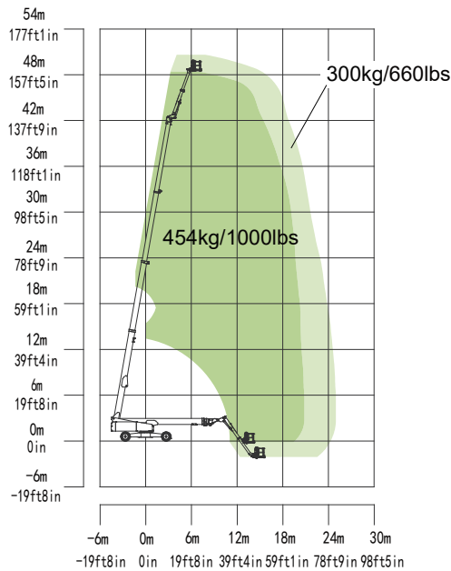
Диаграмма рабочей зоны ZT51J
